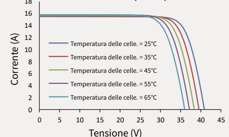
Corrente-Tensione (510W)
