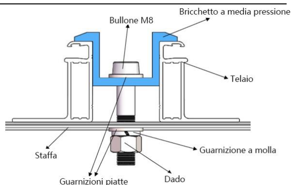
Fig. 12 Schema di installazione del morsetto centrale
