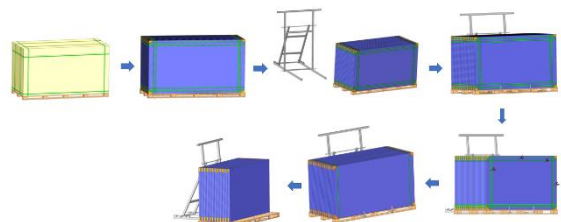
Passaggi per il disimballaggio del pacchetto verticale sul lato corto
