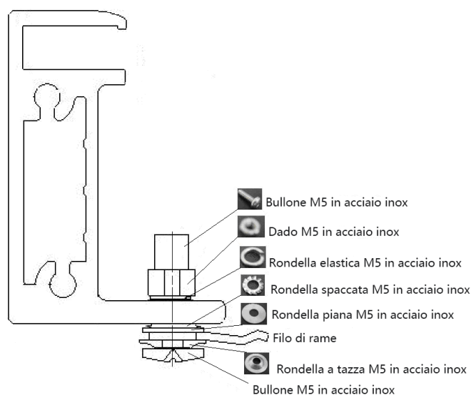
Figura 12 Messa a terra del telaio in alluminio con filo di rame
