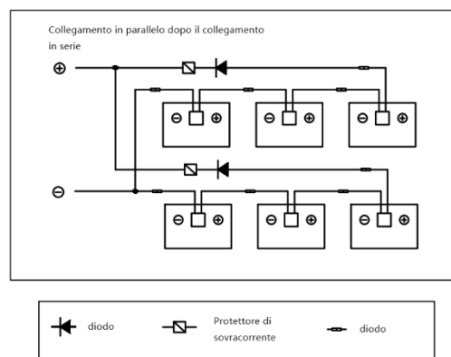
Figura 13 Schema dei collegamenti elettrici
